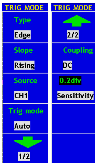
Fig. 33 Edge trigger menu
